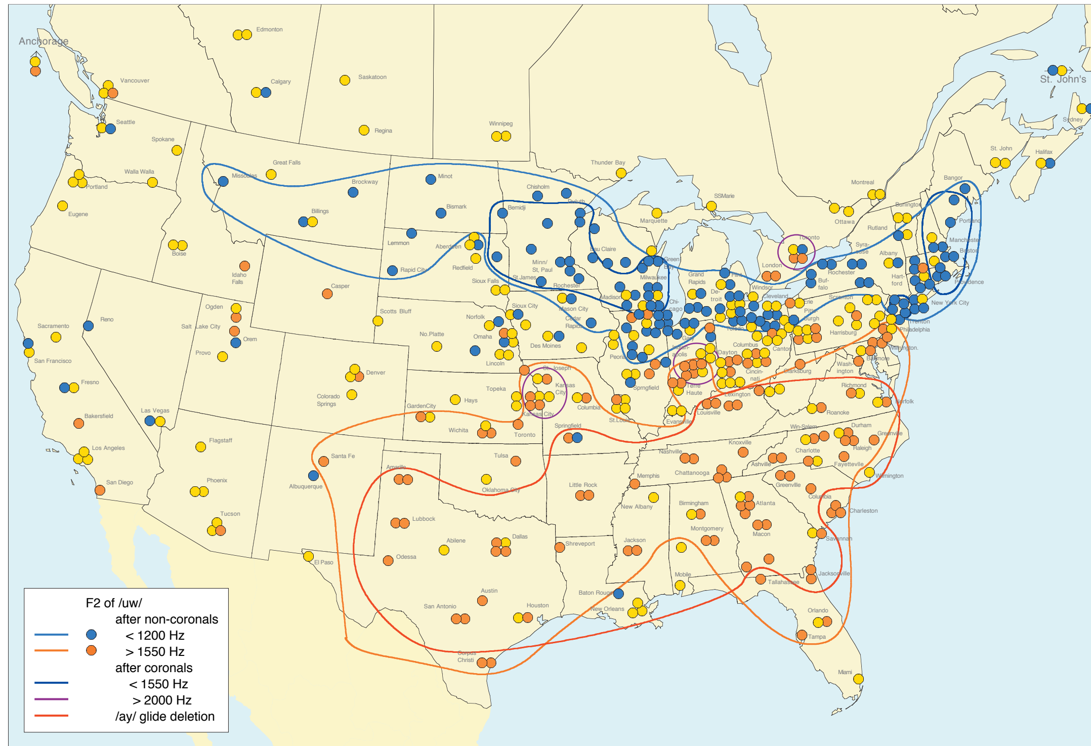
Map 12.2. Fronting of /uw/ after non-coronals (Kuw)
